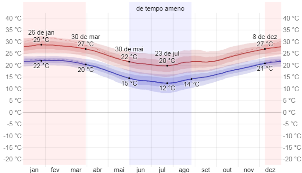
Figura 02 - Temperatura máxima (linha vermelha) e mínima (linha azul) médias, com faixas do 25º ao 75º e do 10º ao 90º percentil. As linhas finas pontilhadas são as temperaturas médias percebidas correspondentes.
